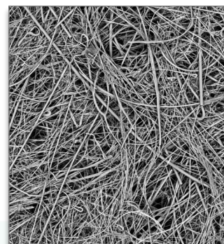
FilterGLA: fotografia al microscopio elettronico
