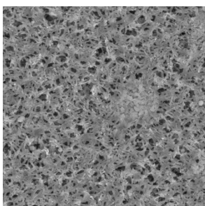
Membrana NYL: fotografia al microscopio elettronico
